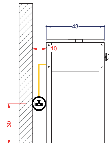
Vista Izquierda
